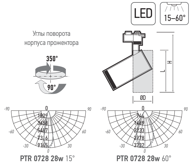
Маркировка угла светораспределения
