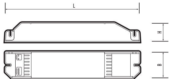
PEPP40-1.0H IP20. (Габаритные размеры)
