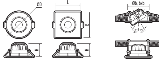
Схема установки PSP-R, PSP-S
